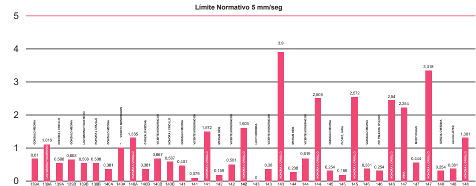
Grafica 2. Resultados Monitoreo Vibración en Evento de Voladura 2024.
