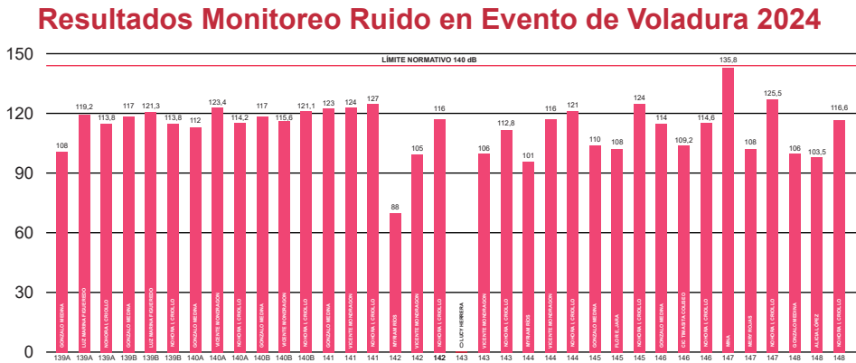
Grafica 1. Resultados Monitoreo Ruido en Evento de Voladura 2024.
