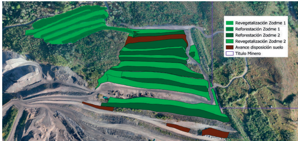
Recuperación Ambiental ZODME's No. 1 y No. 2 proyecto "Cantera el Pedregal".
